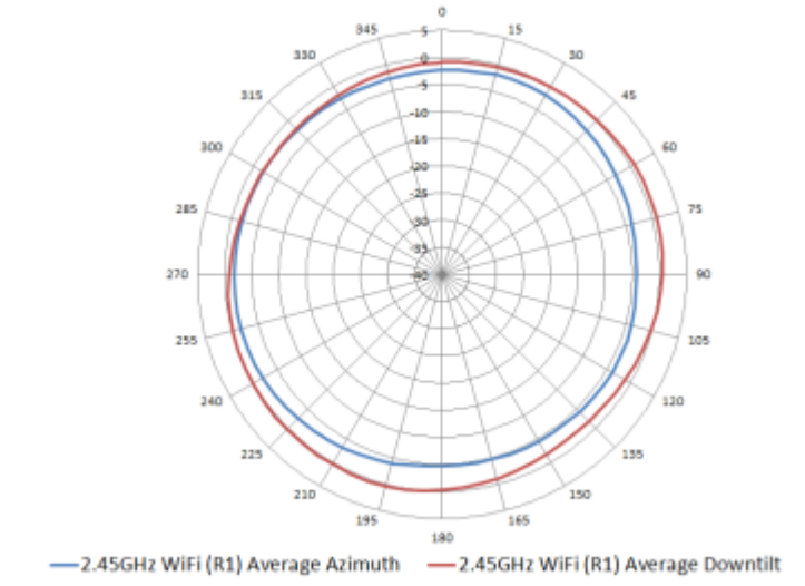
2.45GHz Wi-Fi (antennas 1, 2)
